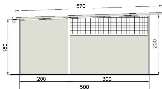
PROSPETTO LATERALE
